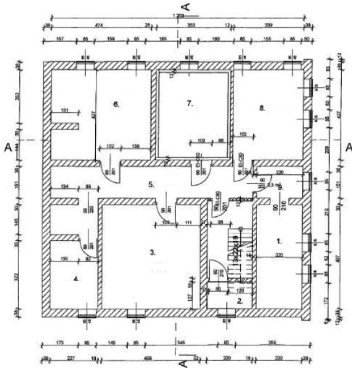
RZUT PIWNICY
